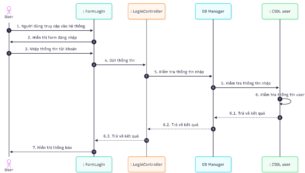
Hình 2.6: Sơ đồ trình tự chức năng “Đăng nhập”
